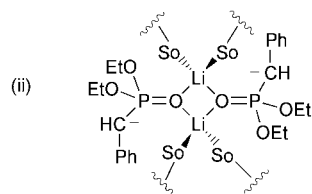
8 : So = DABCO
