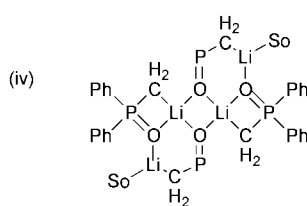
10 : So = TMEDA
