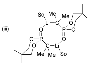
9 : So = TMEDA
